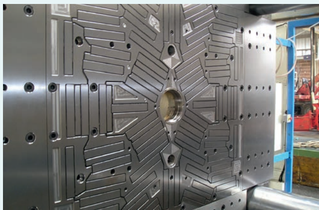
Pressmag HP auf einer 32000 kN Maschine
